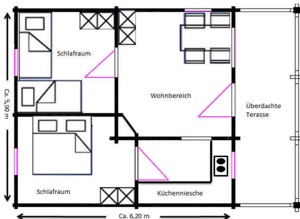
Mustergrundriss Blockhütten 3,4,5,6,7 und 8 (Abweichende Bettenaufteilung beachten)
